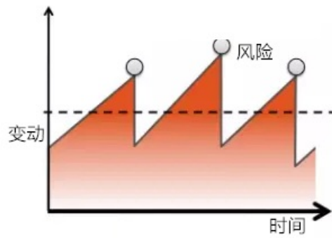
瀑布模式
